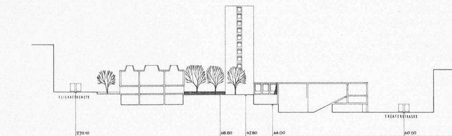
SCHNITT II
