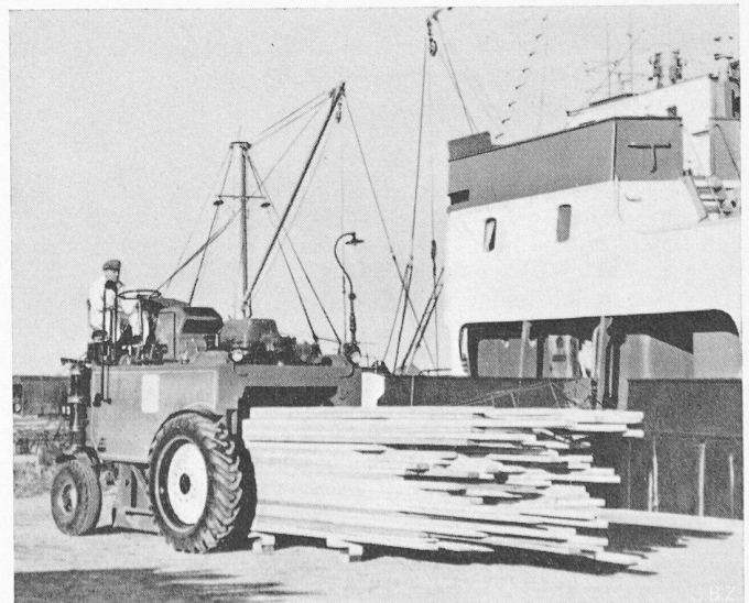
Der Klemmgriff-Lastenträger «Timber-Wolf»
