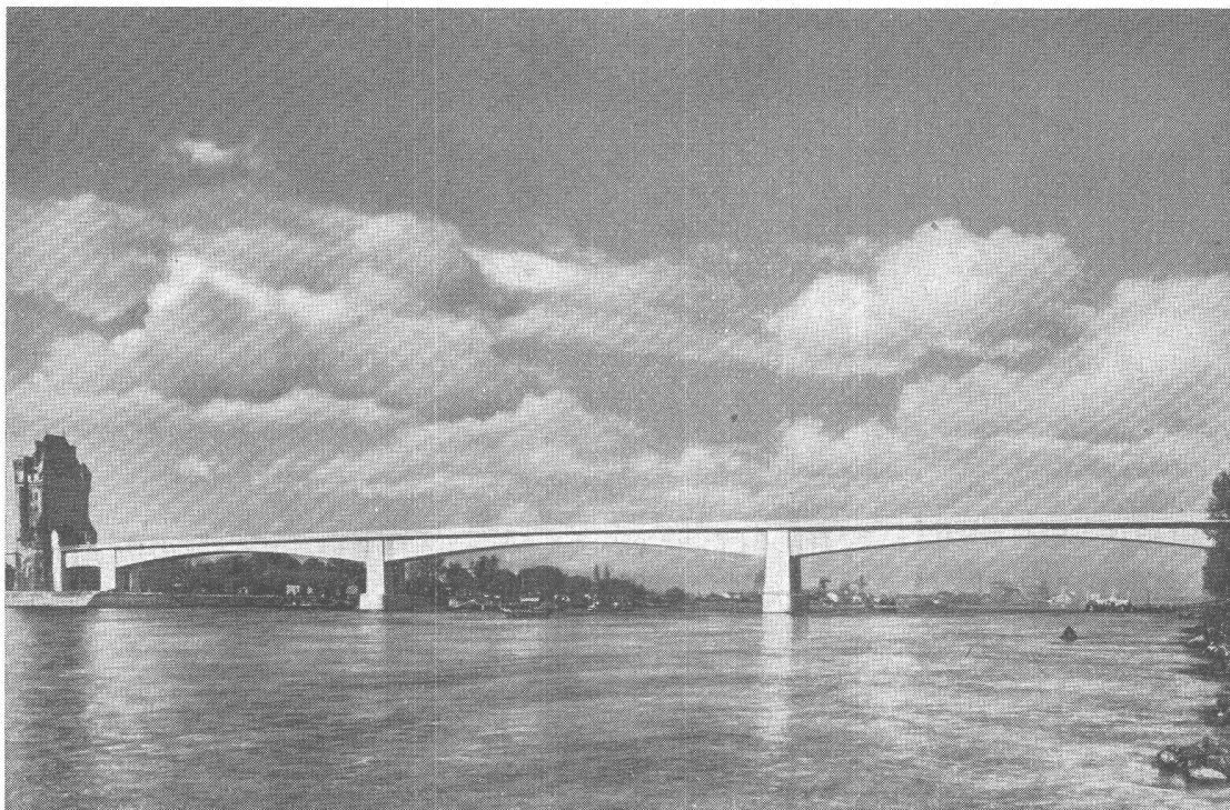
Nibelungenbrücke in Worms: Vorspannbeton, ausgeführt durch Dyckerhof und Widmann, mit PLASTIMENT-Zusatz
