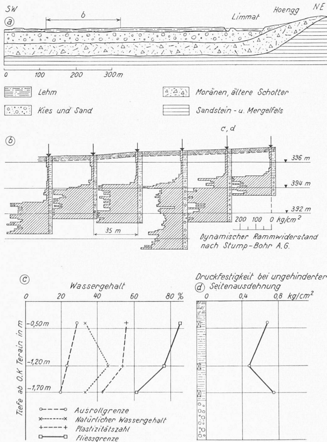
Bild 18. Generelles geologisches Querprofil (a), Sondier- (b) und Laboratoriumsresultate (c, d) aus dem Limmattal (südwestlich der Höngrgerbrücke) unterhalb Zürich
