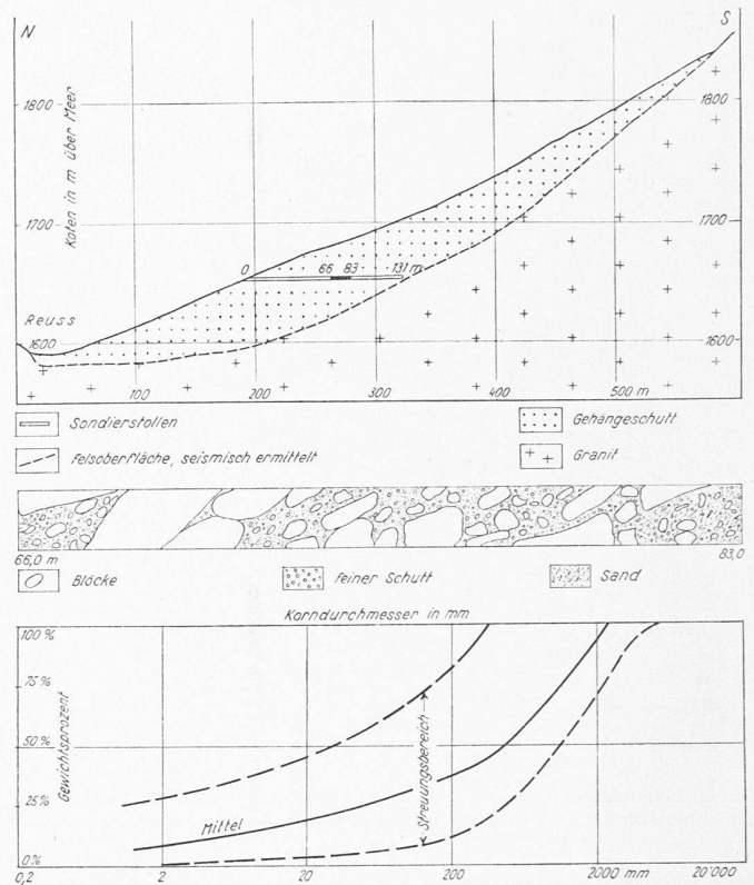
Bild 12. Gehängeschuttkegel Göschenalp, generelles geologisches Querprofil, Stollenaufnahme und Kornverteilung des Stollenmaterials. Nach Unterlagen der Elektrowatt AG.
