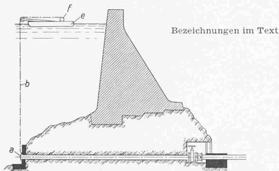
Bild 1. Speicherwerk mit Notverschluss in grösserer Tiefe
