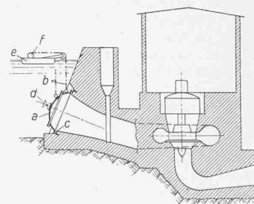
Bild 3. Flusswerk mit Notverschluss
