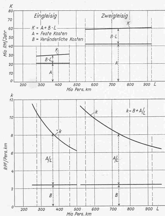
Bild 7. Gesamtkosten K in Mio RM/Jahr und spezifizierten Kosten k in RPF/Pers. km in Abhängigkeit der Verkehrsleistung
