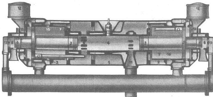
Schnittbild eines 2stufigen Junkers-Freikolben-Dieselskompressors
