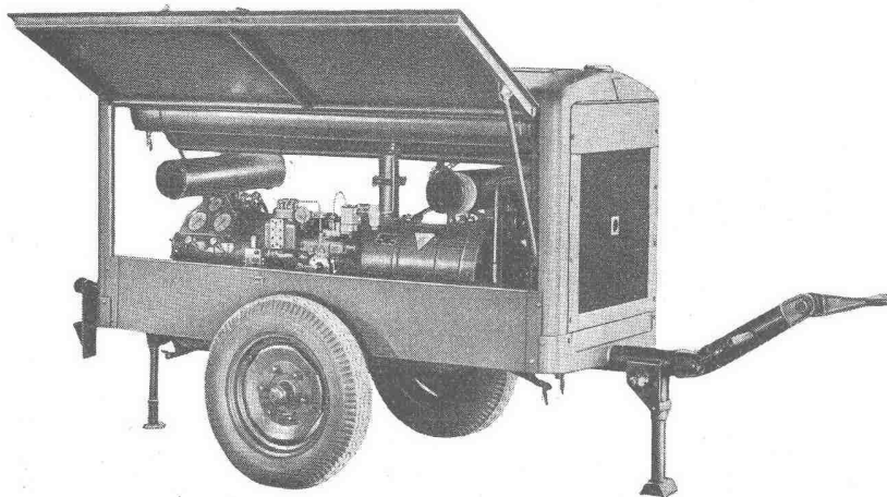
Typ 2 FK 115 A, fahrbar, für 2—3 Hämmer
