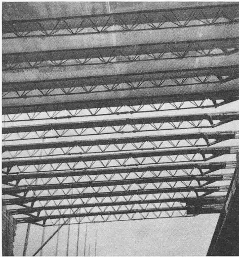
Bild 10. Hico Schalungsträger
