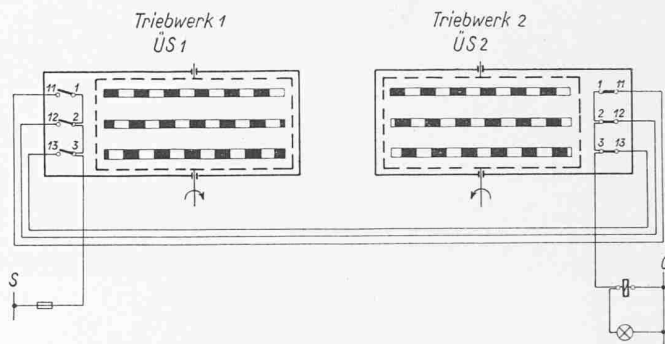
Bild 24. Schaltung zur Gleichlaufüberwachung der Windwerkmotoren
