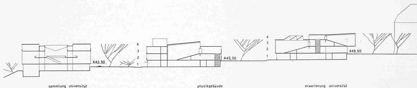
Längsschnitt Südost-Nordwest
