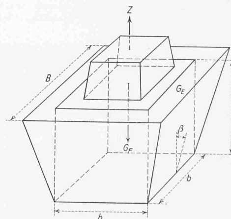
Bild 2. Berechnung der Einzelfundamente nach der Methode des Pyramidenstumpfs.
