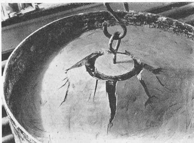
Bild 6. Modellfundament unmittelbar vor dem Bruch
