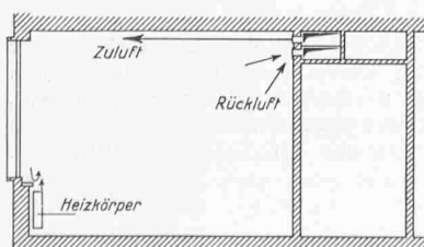
Bild 1. Belüftung eines Büraumes durch Luftkanäle (konventionelles System)
