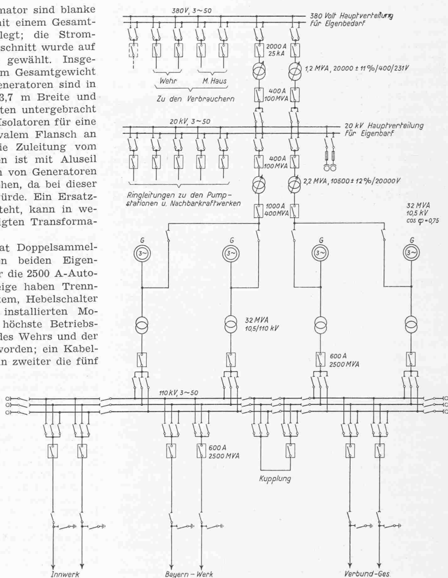
Bild 51. Vereinfachtes Schaltschema
