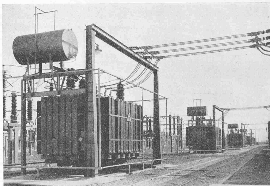
Bild 52. Blocktransformatoren in der 110 kV-Schaltanlage
