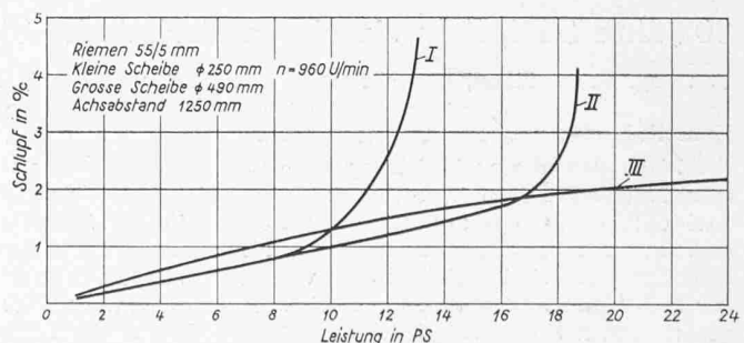
Bild 12. Durch Messung ermittelter Schlupf I und II an gewöhnlichem Riemenantrieb, III an Sespa-Antrieb. Bei I und II ausgeprägte Belastungsgrenze durch beginnendes Gleiten, bei III ohne Belastungsgrenze
