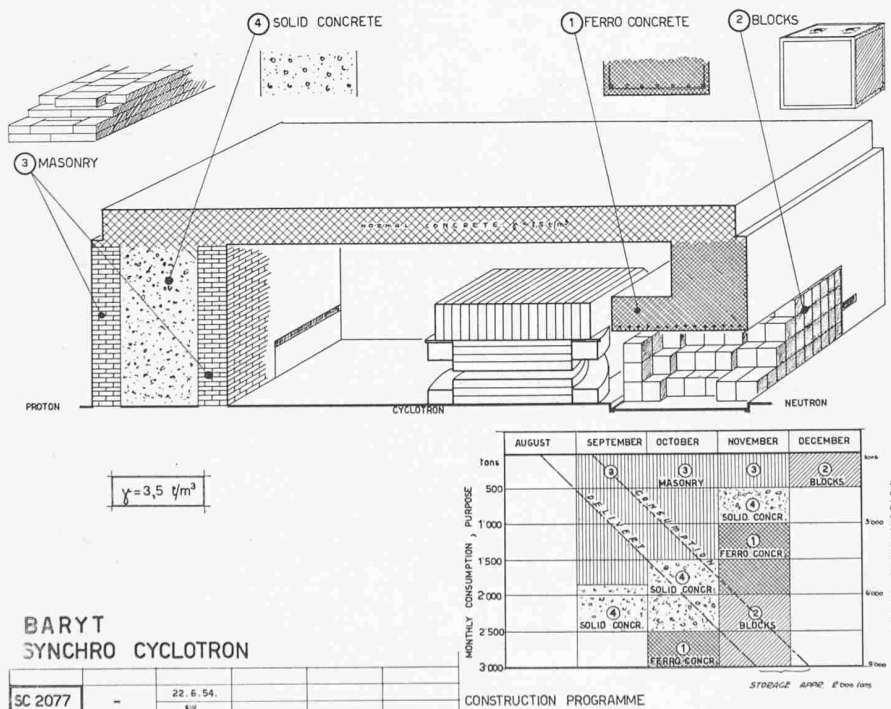
Fig. 12. Etudes concernant la confection de béton lourd à base de baryte (densité 3,5) contre le rayonnement dangereux
