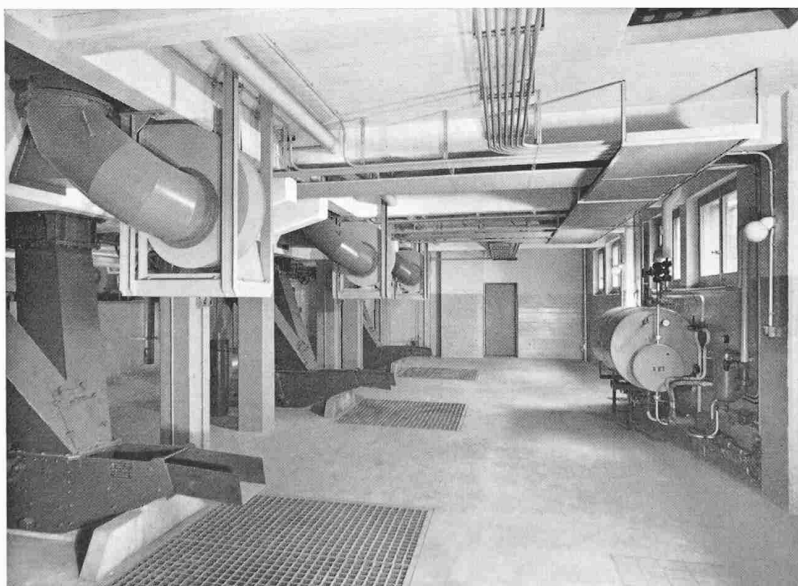
Unterwindventilatoren und Halbbrassentschlacker im Geschoss B des Kesselhauses, rechts Brennölversorgungsinstallation
