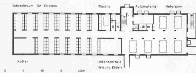
Bild 40. Keller
