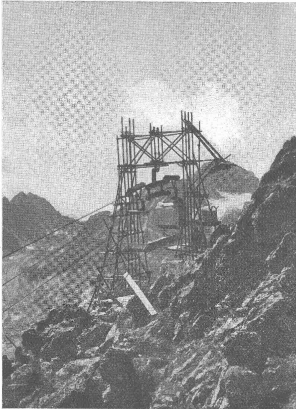
Provisorischer Portalmaß für Seilbahn Corviglia-Piz Nair 2800 m ü.M. August 1953
