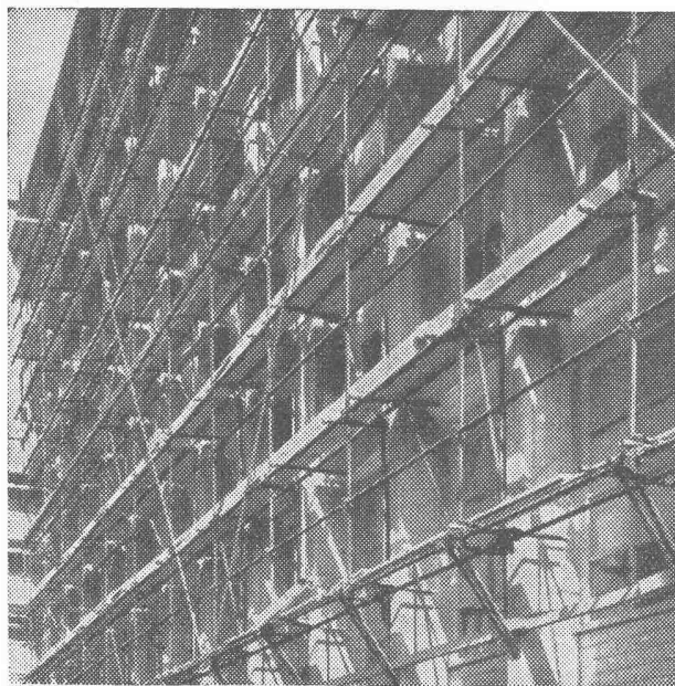
ACROW - Rohrgerüste
