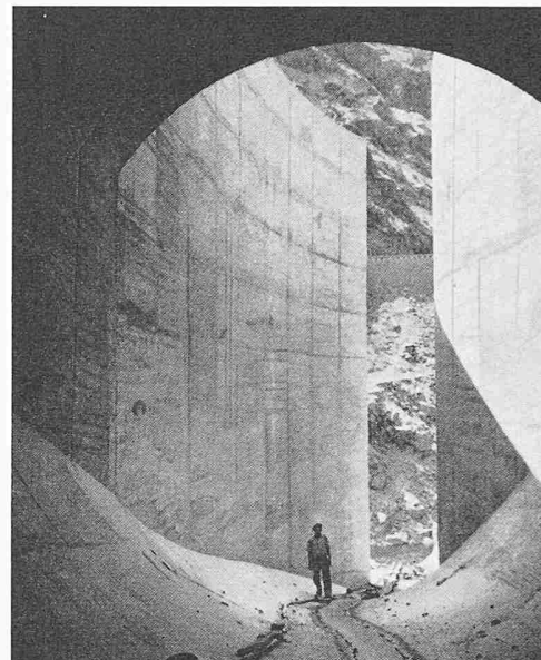
Bild 3. Auslauf des Hochwasserüberlaufes links. Uebergang aus Kreisprofil \varnothing 6,5 m in vertikales Rechteck
