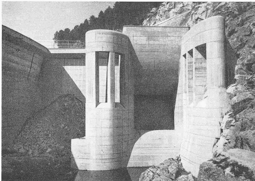
Bild 2. Einlauf zum Hochwasser-Ueberlauf rechts
