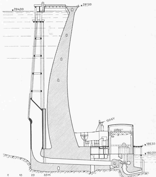
Bild 5. Querschnitt des Kraftwerkes, Masstab 1:1400
