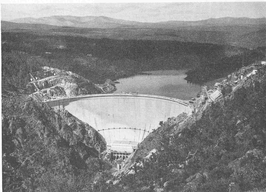
Bild 1. Ansicht des Kraftwerkes Cabril im März 1954. Am Berghang rechts der Werkplatz, links die Bahnhöfe von oben drei, unten einem Kabelkran. Stausee auf Kote 250 (Normalstau 294)
