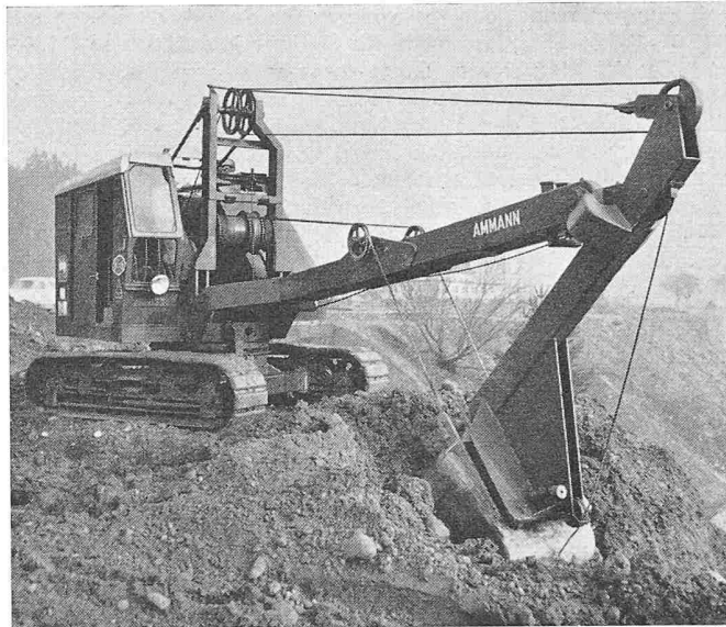
P & H-Raupenbagger mit Tieflöffelausrüstung und Kübel von 600 l Inhalt
