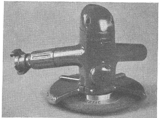
Bild 4. Hochleistungs-Scheibenschleifmaschine S 180
