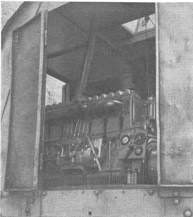
Bild 2. Raupenbagger mit luftgekühltem SLM-Dieselmotor
