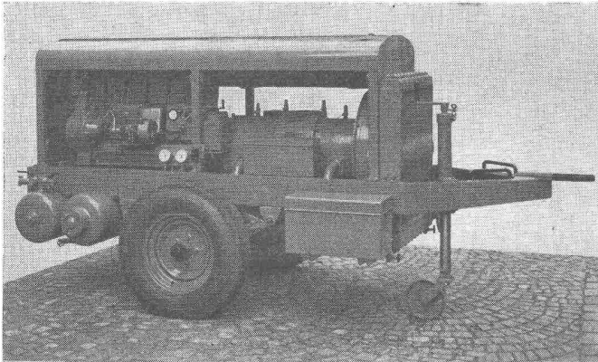
Bild 1. Luftgekühlter, fahrbarer SLM-Rotationskompressor mit luftgekühltem SLM-Dieselmotor
