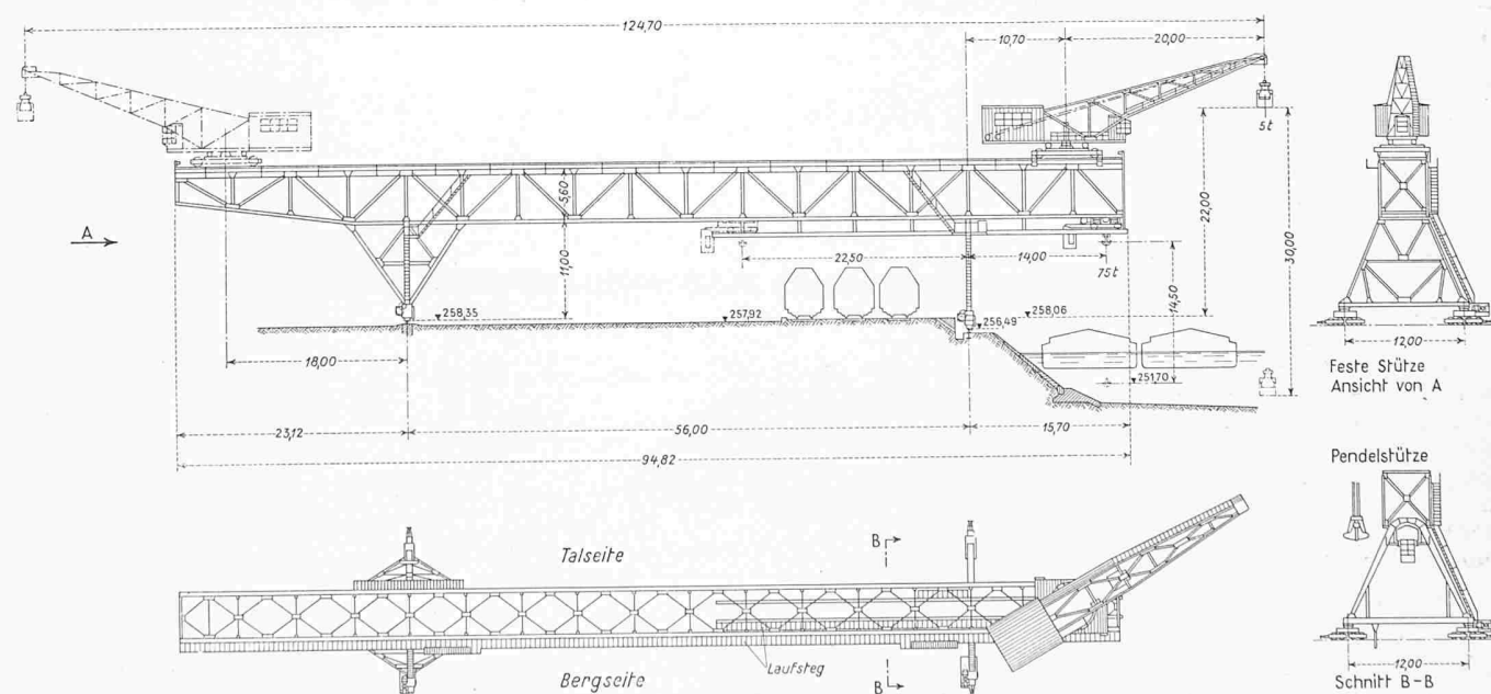
Bild 1. Verladebrücke der Ultra AG. im Auhafen Muttentz, mit Greiferdrehkran von 5 t und 20 m Ausladung und Schwerlastkatze von 75 t (Probelast 90 t). Brückenfahrwerk mit separaten Schemelantrieben. — Masstab 1:800
