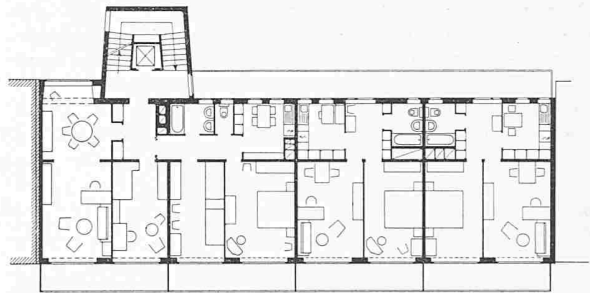
Normalgeschoss (Laubengang an der Nordseite)
