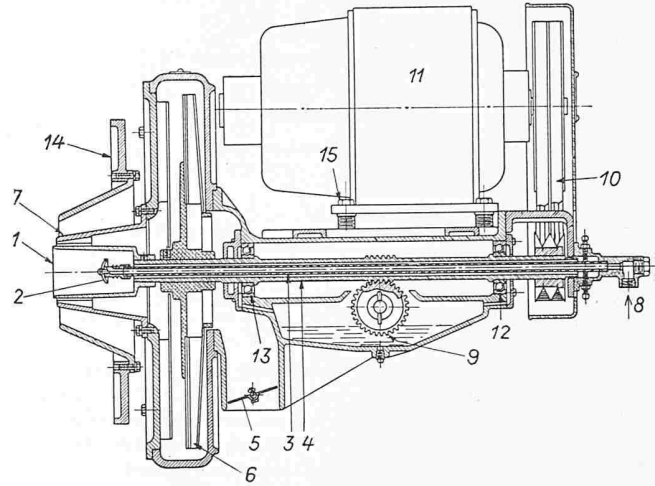
Bild 5. Rotationsbrenner für Schwerölförderung. 1 Zerstäuberbecher, 2 Schirm mit Oelaustritt, 3 feste Oelzuleitung, 4 rotierende Hohlwelle, 5 Luftklappe, 6 Ventilatorrad, 7 Primärluft-Konus, 8 Oelzufuhr, 9 Schneckengetriebe für Oelpumpenantrieb, 10 Keilriementrieb, 11 Elektromotor, 12 hinteres Kugellager zu 4, 13 vorderes Kugellager zu 4, 14 Flanschring zum Befestigen des Brenners an der Kesselfront, 15 Schrauben zum Spannen des Keilriemens.
