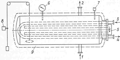
Bild 4. Heizölvorwärmer. 1 Eintritt des kalten Oels, 2 Austritt des warmen Oels, 3 Heisswasser-Vorlauf, 4 Heisswasser-Rücklauf, 5 elektrischer Heizsatz, 6 Oelthermometer, 7 Thermostat, 8 Schwimmerschalter für Pumpensteuerung, 9 Isolierung.
