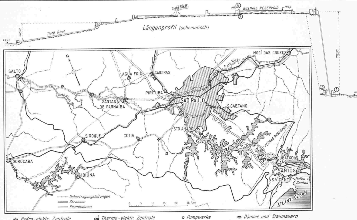
Bild 40. Energieerzeugungsanlagen in der Zone Sao Paulo - Santos, Uebersicht 1:900 000 und Längenprofil. Die Zahlen in Kreisen beziehen sich auf die Bilder 41, 43 und 44.
