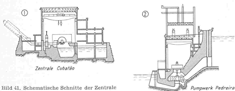
Bild 41. Schematische Schnitte der Zentrale Cubatão und des Pumpwerks Pedreira
