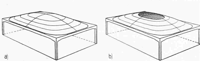
Bilder 4a und 4b. Grundformen der Einzelschale auf vier Eckstützen
