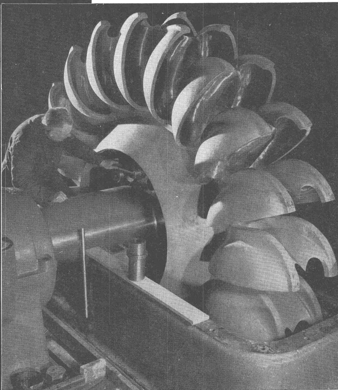
Centrale de Gondo, Roue Pelton de 22 600 ch
