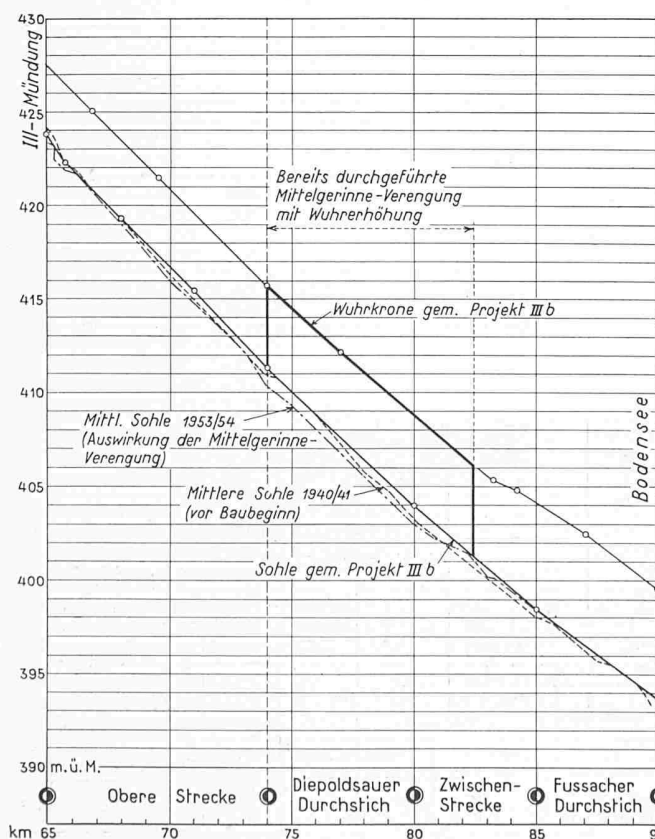
Bild 8. Sohlenlage und Höhe der Mittelgerinne - Wührkrone gemäss Projekt III b.
