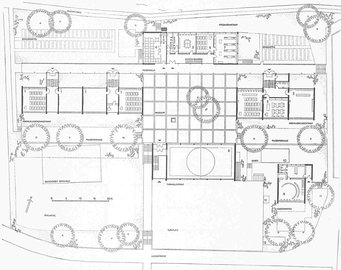
Primarschulhaus im Sömmmerli-Feldli, Erdgeschossgrundriss 1:650. Legende: 1 Klassenzimmer, 2 Werkklassen Mädchen, 3 Handarbeitszimmer Mädchen, 4 Hort, 5 Lehrerzimmer, 6 Theoriezimmer, 7 Schulküche, 8 Turnhalle, 9 Kindergarten
