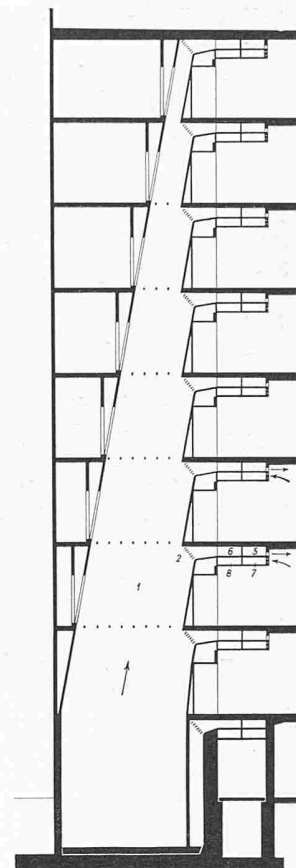
Bild 12. Vertikalschacht für Zuluft 1:200
