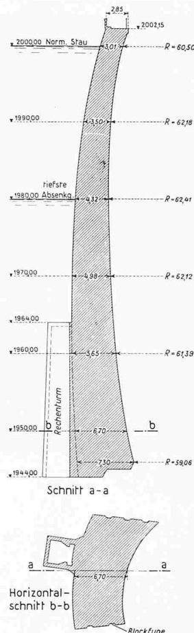
Bild 5. Möllsperre, Querschnitt 1:650
