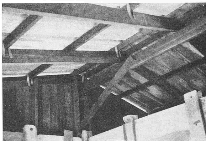
Bild 9. Dachkonstruktion
