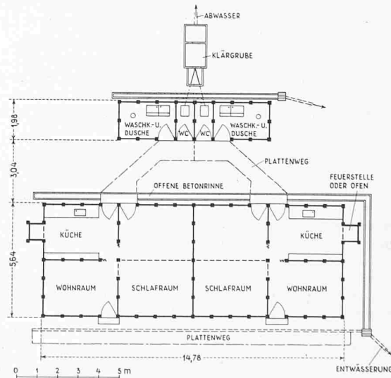
Bild 5. Grundriss einer Zweifamilieneinheit 1:250
