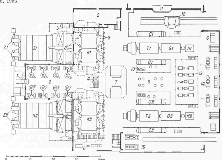
Bild 1. Grundriss einer Kraftzentrale mit zwei Block-Einheiten und zentral gelegener Warte, von der aus beide Einheiten (je ein Kessel und eine Turbine) gesteuert und überwacht werden.
