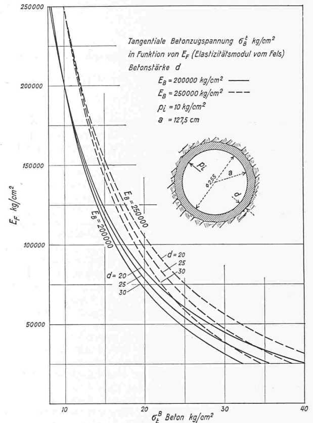
Bild 3. Tangentialen Betonzugspannung der Betonauskleidung
