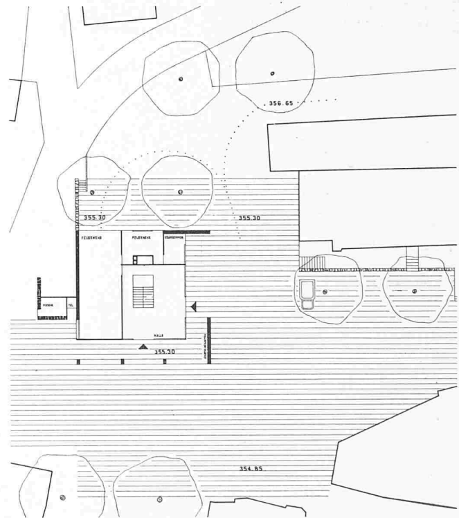
Erdgeschoss Masstab 1:600
