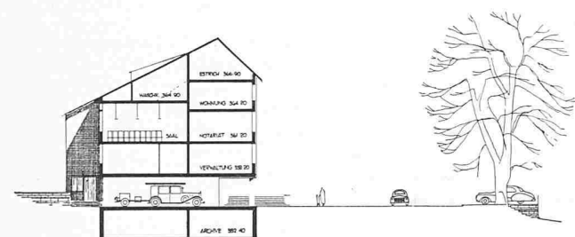
Schnitt
