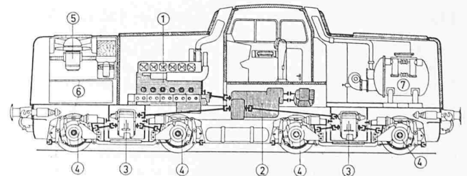
Bild 1. Kraus-Maffei-Diesellokomotive V 80 von 1000 PS mit hydraulischer Kraftübertragung und Gelenkwellenantrieb. 1 Dieselmotor, 2 hydraul. Getriebe, 3 Umschalt- und Verteilergestriebe, 4 Kegellachstrieb, 5 Kühlergruppe, 6 Treibstoffbehälter, 7 Dampfkessel für Zugheizung
