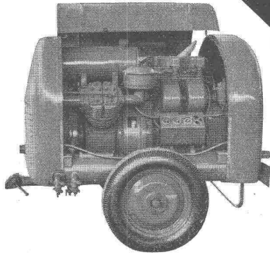
Luftgekühlte Kompressoranlage «robot» DV-20 2 Zylinder 2stufig 2 m 3 /Min. 7 atü 4 Typen ortsfest und fahrbar mit Diesel- oder Elektroantrieb
