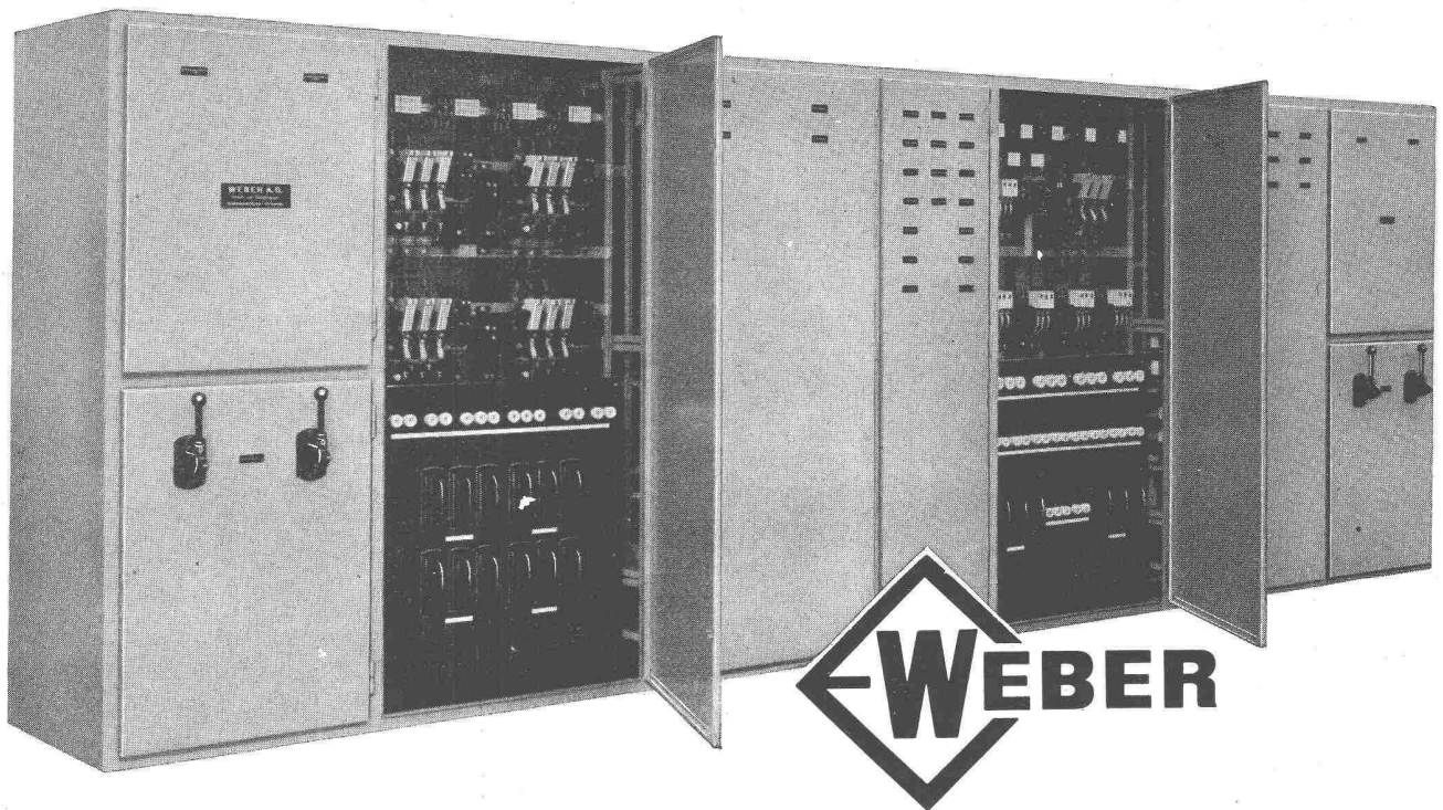
Hauptverteil- und Schützenschrank in staub- und spritzwasserdichter Ausführung, für einen Papiermaschinen-Antrieb mit 30 Motoren einer Papierfabrik.
