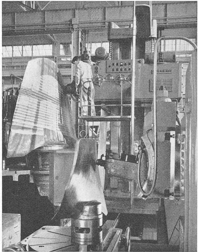
Bild 11. Elektronisch gesteuerte Kopierfräsmaschine, die bei Escher Wyss entwickelt und gebaut wurde. Im Vordergrund das von Hand gearbeitete Modell einer Kaplanturbinenschaufel, das von einer Fühlereinrichtung abgetastet wird. Die Bewegungen werden automatisch vergrössert auf den Fräser übertragen.
