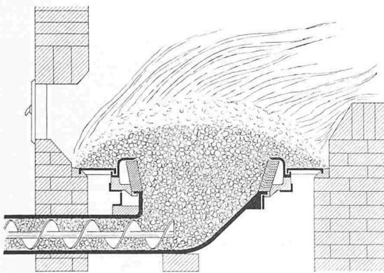
Bild 3. Mechanische Unterschubfeuerung
