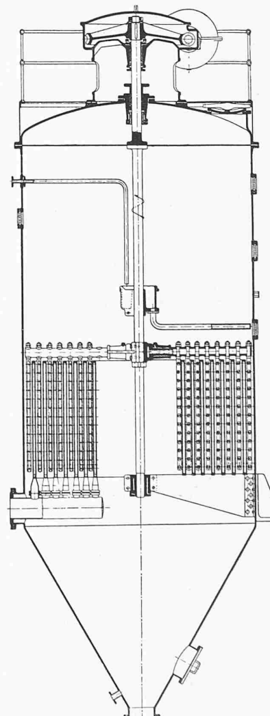
Bild 8. Sole-Eindampfungsapparat mit Ringheizkörper und Abstreifer der Anlage in Reichenhall nach Bild 7
