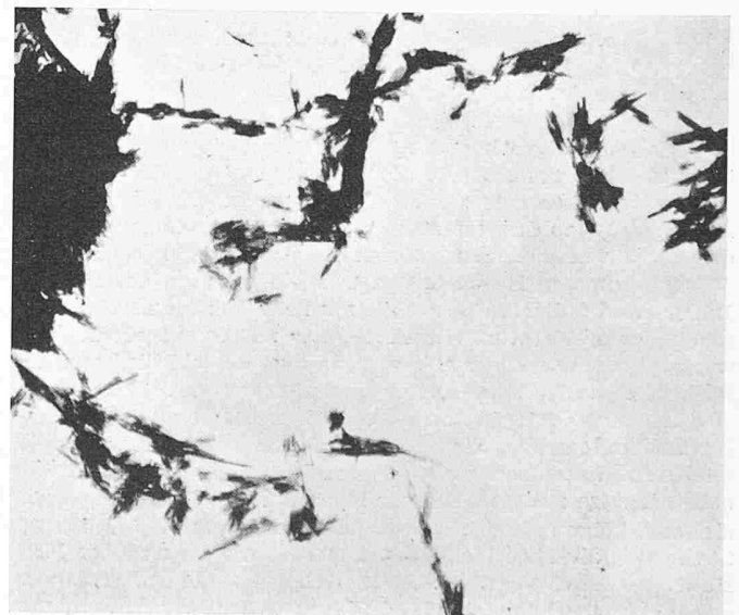
Bild 5. Synthetischer Chrysotilasbest. Elektronenmikroskopische Aufnahme bei 9000facher Vergrösserung. Haufwerk kleinster Kristalle
