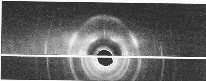
Bild 3. Röntgenanalytisches Faserdiagramm eines natürlichen Chrysotils (oben) und Pulverdiagramm nach Debye-Scherrer eines synthetischen Chrysotils (unten)
