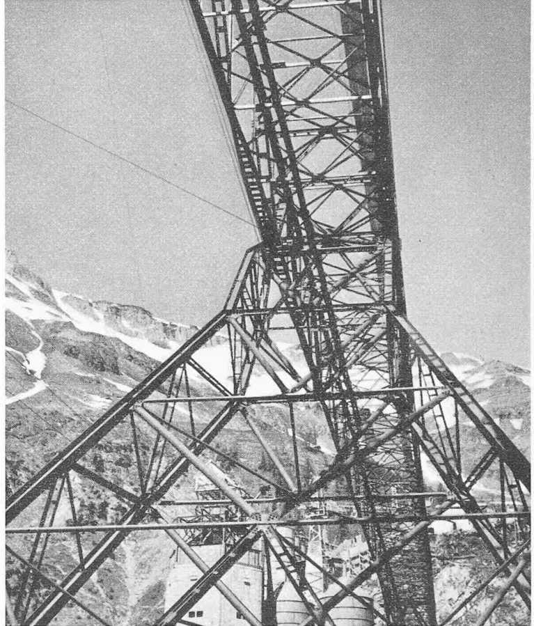
Bild 7. Draufsicht auf den Kämpferbock (rechtes Ufer, hinten Felswand auf dem linken Ufer)
