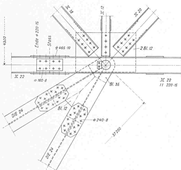
Bild 5. Knotenpunkt am Stützenkopf, Masstab 1:30
