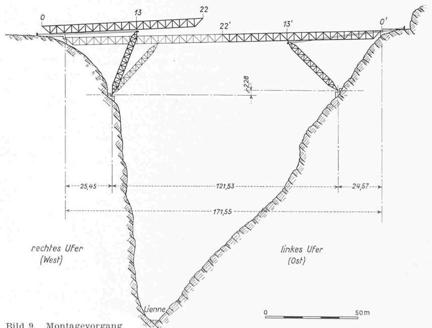
Bild 9. Montagevorgang
