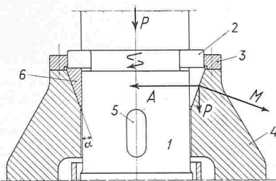
Fig. 6. Schéma de principe d'un manchon de pivoterie avec dispositif anti-rouille d'appui
