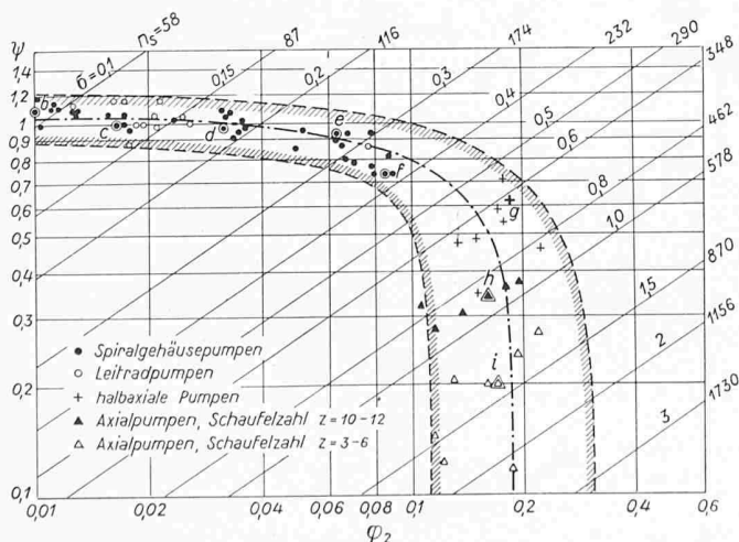
Bild 7. Druckziffer, Durchflussziffer und spezifische Schnellläufigkeit für verschiedenartige Kreispumpen
