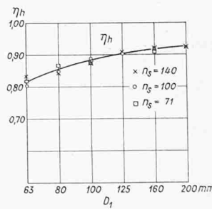
Bild 3 b. \eta_h in Funktion des Laufradinnendurchmessers D_1
