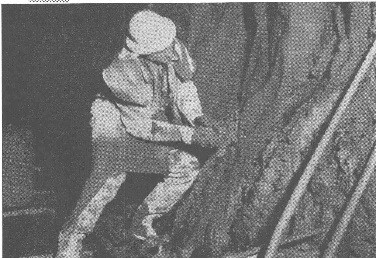
Maggia-Kraftwerke AG., Locarno. Vordichtung des Druckstollens Galleria-Verbano mit BARRA- RAPID U.
