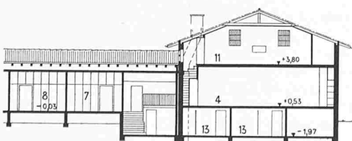
SCHNITT A-A
