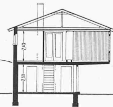
SNITT
