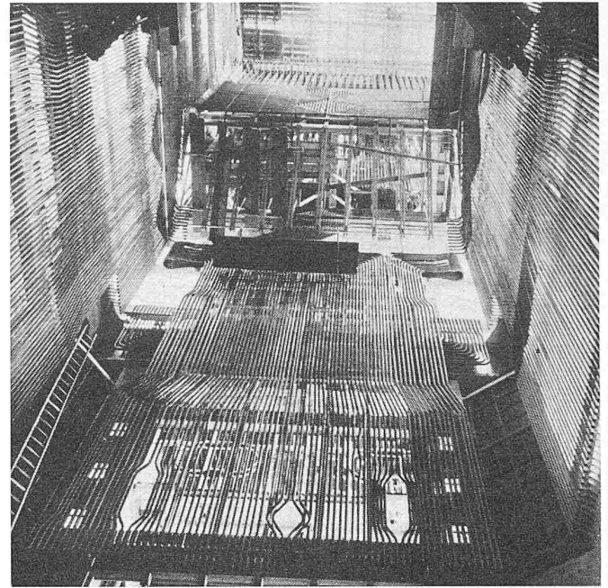
Bild 30. Blick in die Brennkammer des Dampferzeugers der Anlage nach Bild 19 von unten gegen die Decke, während der Montage
